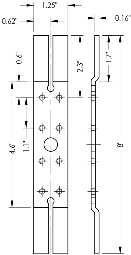
22 DOOR HINGE REINFORCEMENT
